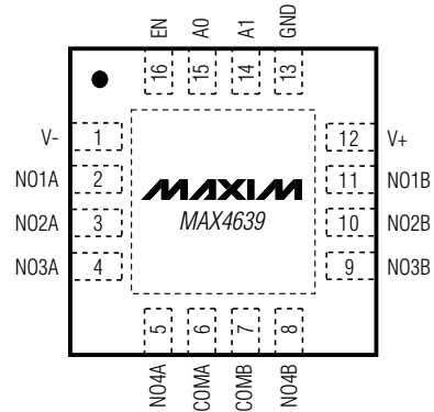
THIN QFN
