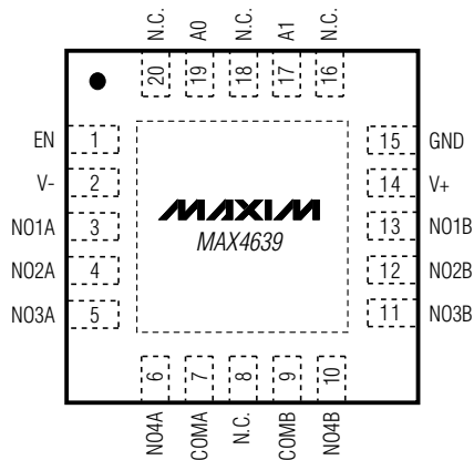
THIN QFN
