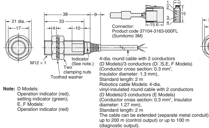
Fig. 8 : E2E-X3D□-N E2E-X2E□/F□
