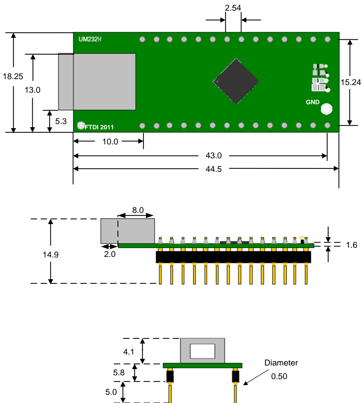
Figure 5.1 : UM232H Module Dimensions
