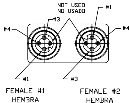
BACK VIEW VISTA TRASERA CONECTORES HEMBRA
