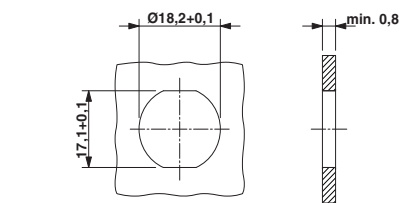
Einbaumaße: ST-E.1N8A6100S, Bohrung mit Verdrehenschutz und Kontermutter (Empfehlung bei Einbau in Stahlblechwand)
