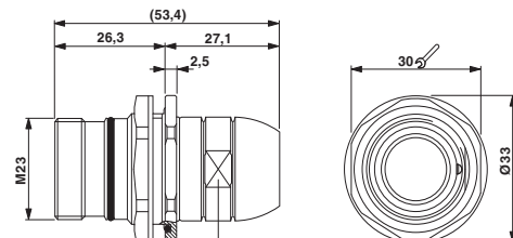
RC-0000000Q0FZ O-Ring axial
