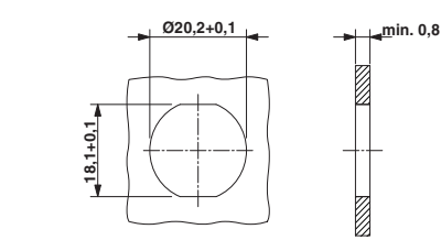
Einbaumaße: ST-E.1N8AH100S, Bohrung mit Verdrehenschutz und Kontermutter (Empfehlung bei Einbau in Stahlblechwand)
