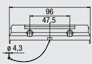
Baugröße 6/size 6
