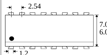
TLP620-4
