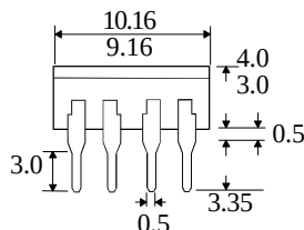
TLP620-4
