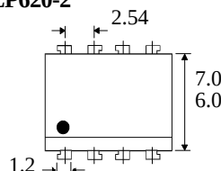
TLP620-2
