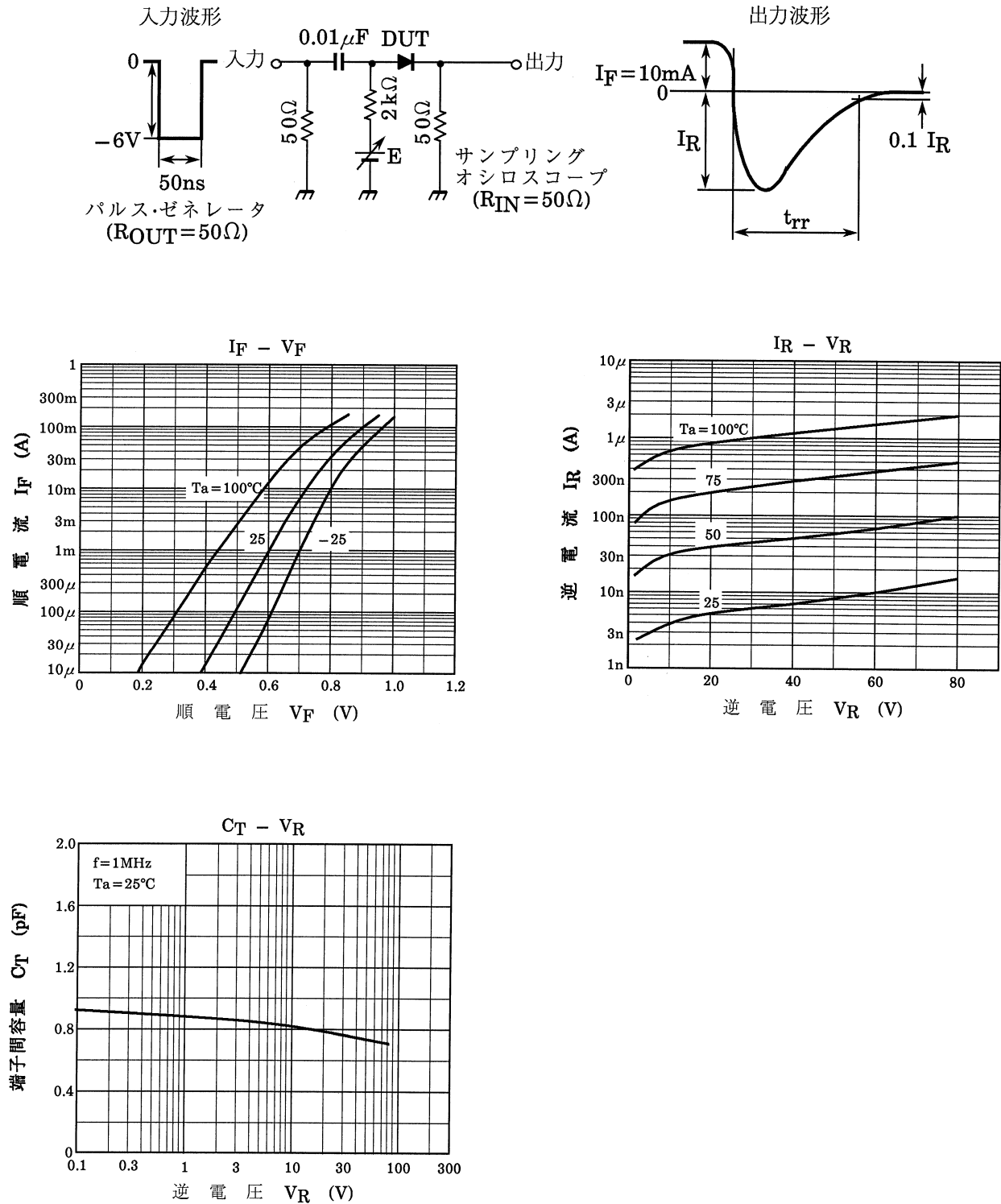
図 1. 逆回復時間 ( t_{rr} ) 測定回路
