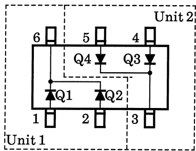
内部接続 (TOP VIEW)
