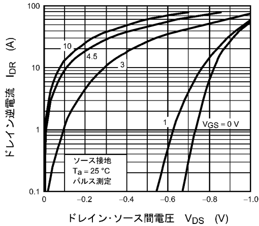
図 8.7 I_{DR} - V_{DS}
