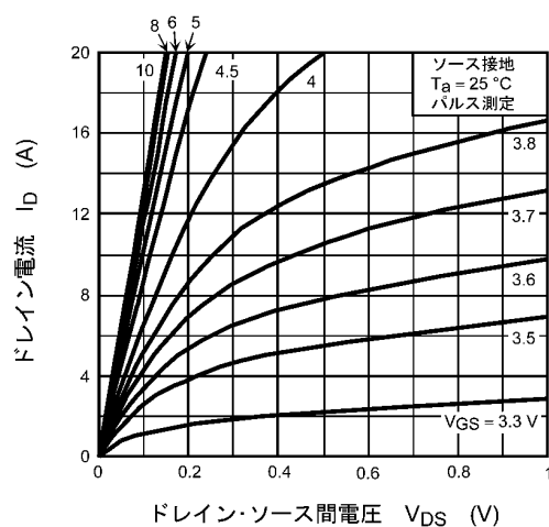
図 8.1 I_D - V_{DS}
