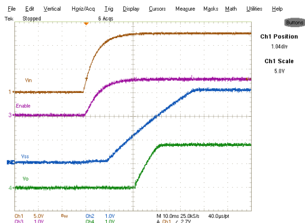
Fig.14: Start-up sequence into 60A load. Ch 1 : V_{in} , Ch 2 : V_{ss} , Ch 3 : Enable, Ch 4 : V_o
