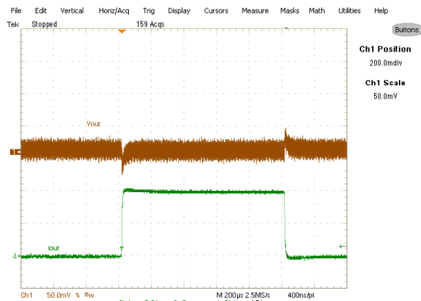
Fig.17: Transient response. Ch 1 : V_o , Ch 4 : I_o (0-10A)
