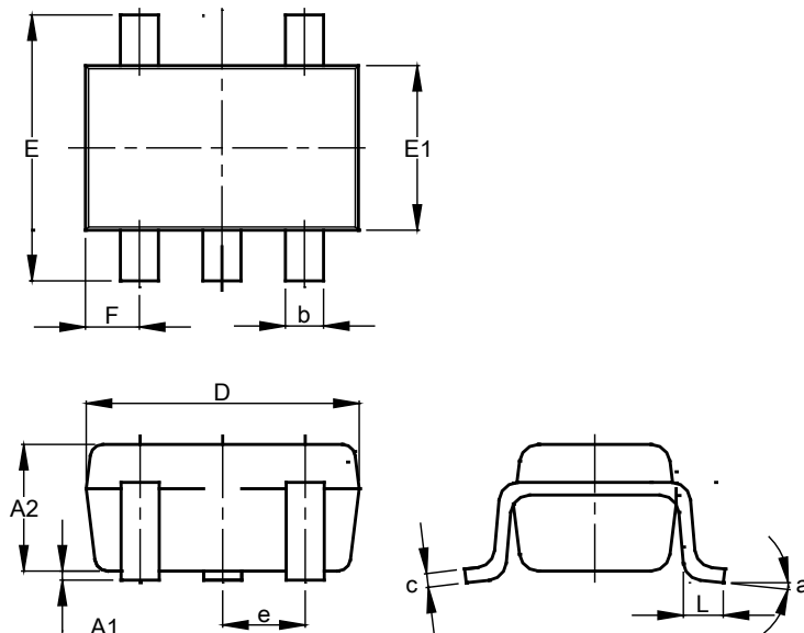
SOT353
