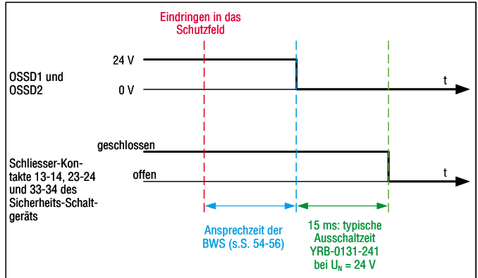
FIG. 39: SCHALTABLAUF DES SICHERHEITS-SCHALTGERÄTS
