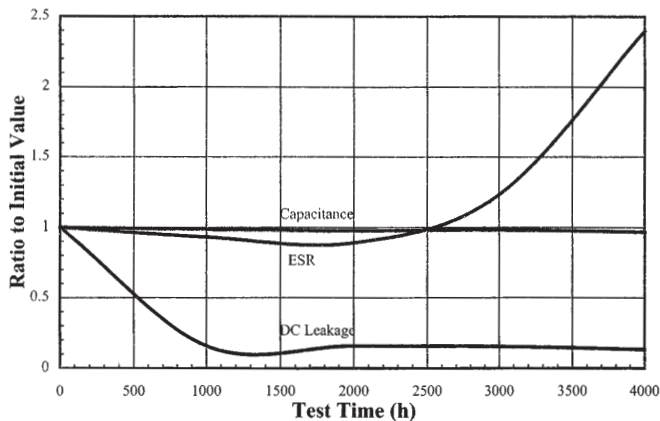
Life Test 150 \mu\text{F} 16 V 105 °C, 556151U016DD2
