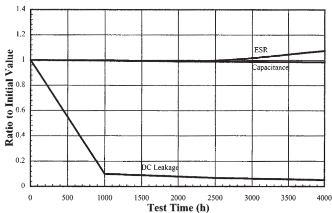
Life Test 10 \mu\text{F} 150 V 105 °C, 556100U150DD2
