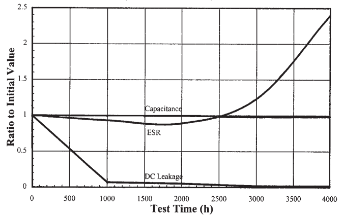
Life Test 50 \mu\text{F} 50 V 105 °C, 556500U050DD2
