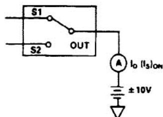
b. AD7592
