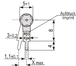
Type 290-1... 298-1
