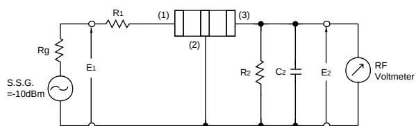
SFECV10M7_A00-R0
