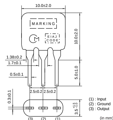
SFKLF10M7NL00-B0
