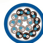
Schnittzeichnung
