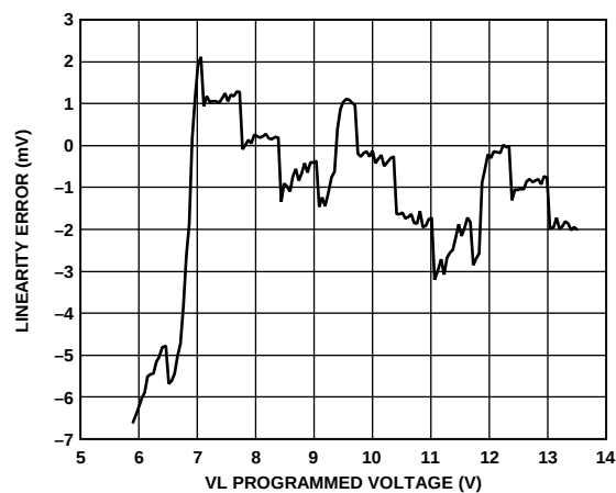
Figure 27. HVOOUT VHH Linearity Error
