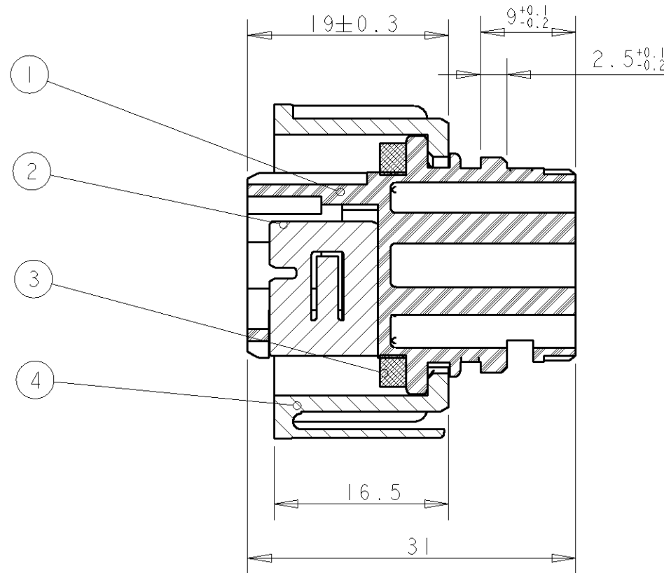
SECTION A-A
