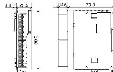
FC4A-N16B1, FC4A-R161
