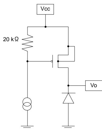
Vo Pin
