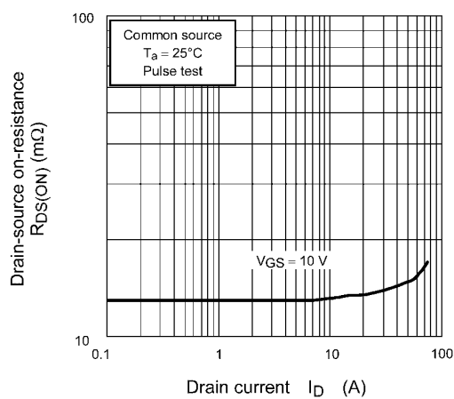
Fig. 8.6 R_{DS(ON)} - I_D
