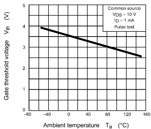
Fig. 8.10 V_{th} - T_a
