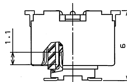
嵌合状態図(参考) (尺度5/1)
