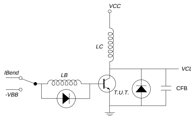
Fig.12. Test Circuit RBSOA. V_{CC} = 150\text{ V} ; -V_{BB} = 1 - 4\text{ V} ; L_C = 1\text{ mH} ; V_{CL} = 1500\text{ V} ; L_B = 0.5 - 2\text{ }\mu\text{H} ; C_{FB} = 1 - 3\text{ nF} ; I_{B(end)} = 0.8 - 4\text{ A}
