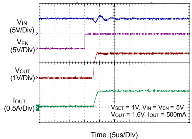
Start Up for EN
