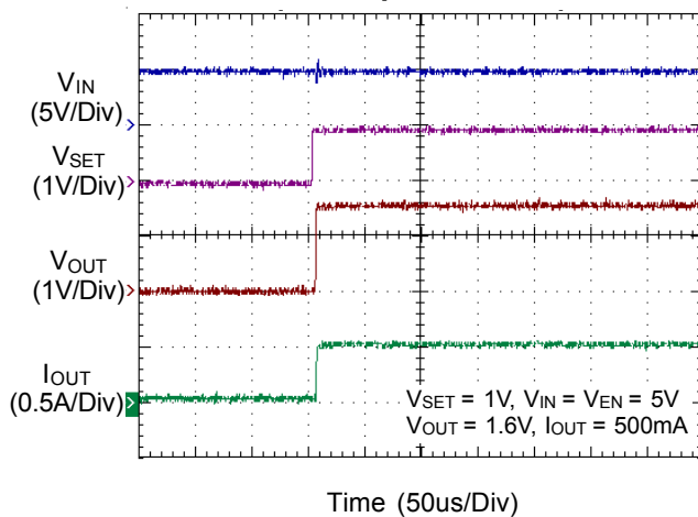
Start Up from VSET
