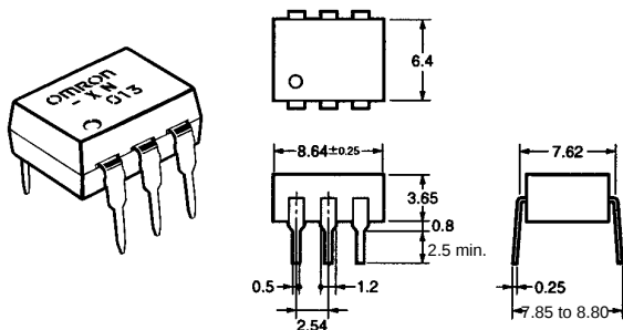
G3VM-XN G3VM-4N
