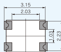
推奨はんだ付けパターン Recommendable soldering pattern (Top view)
