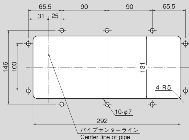
パネル穴明け寸法 Panel drilling dimensions
