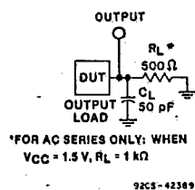
Fig. 5 - Test circuit.
