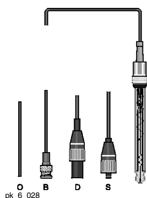
Type PHES 112 FE
