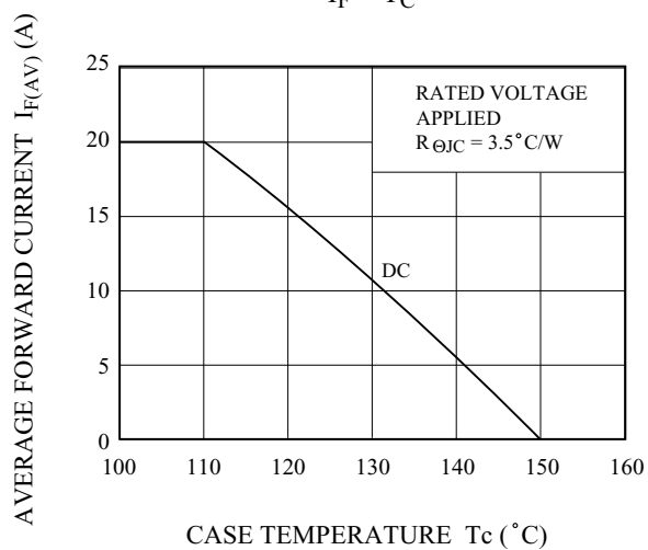
I_F - T_C
