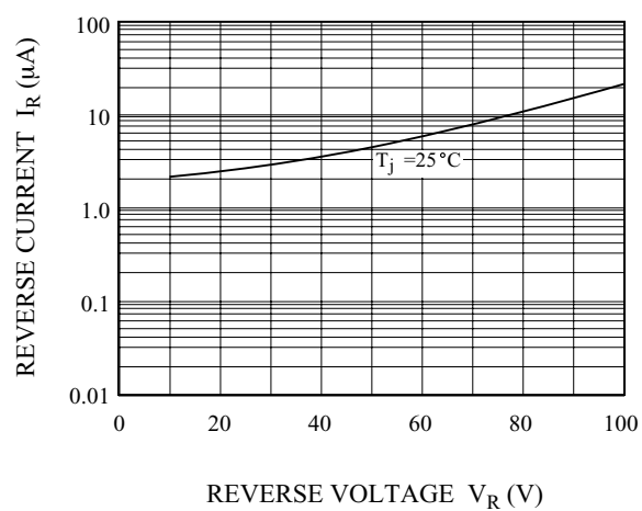
I_R - V_R
