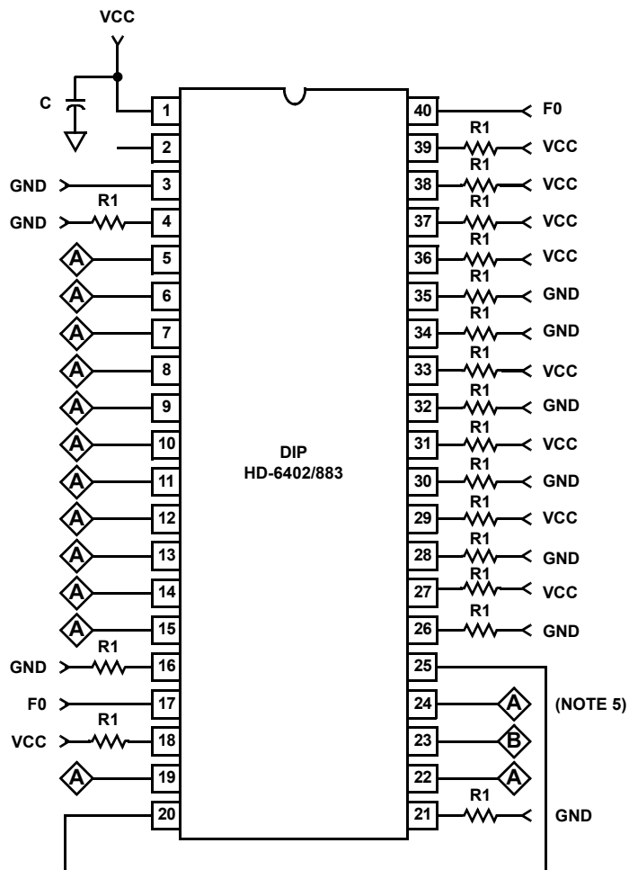
HD-6402/883 CERDIP
