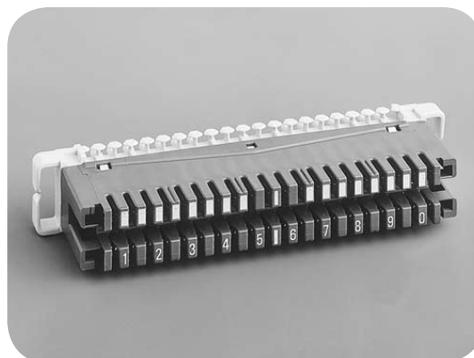
LSA-PLUS®-Schaltleiste 2/10
