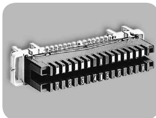
LSA PROFIL®-Schaltleiste 2/8
