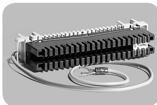
LSA PROFIL®-Erddrahtleiste 2/34
