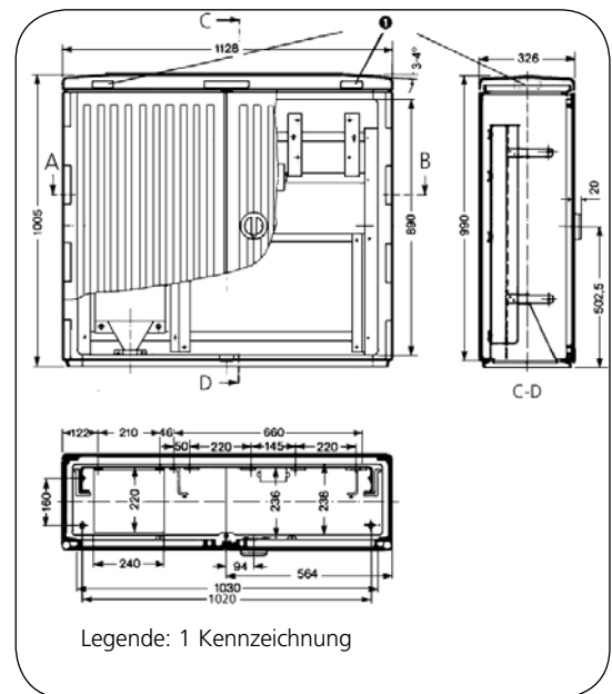
Maßbild Gehäuse 83
