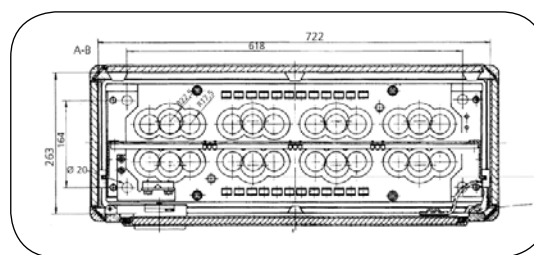
Schnitt-Maßbild: Kabelverzweiger 59m1
