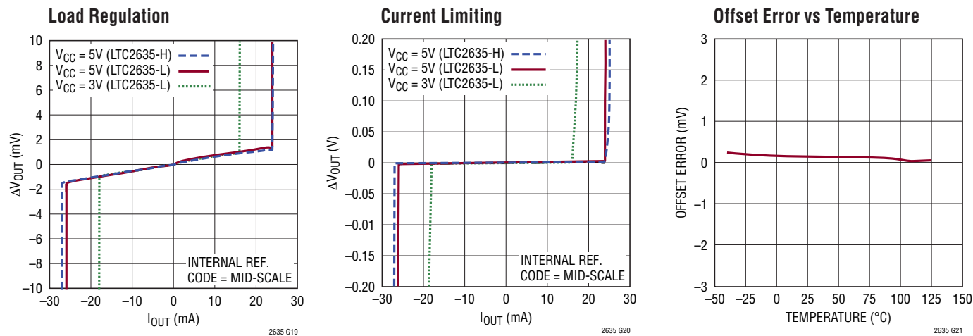
LTC2635
