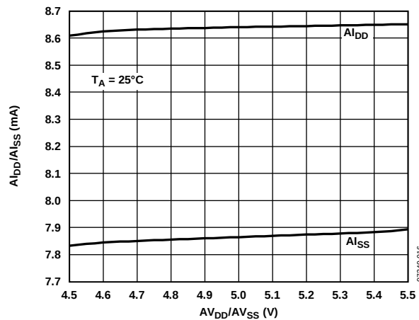
Figure 11. I_{DD}/I_{SS} vs. AV_{DD}/AV_{SS}
