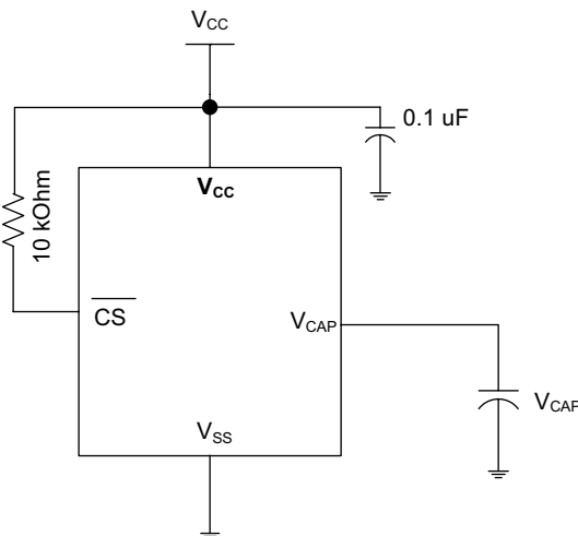
Figure 3. AutoStore Mode
