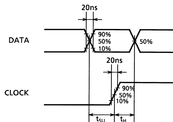
波形 3
