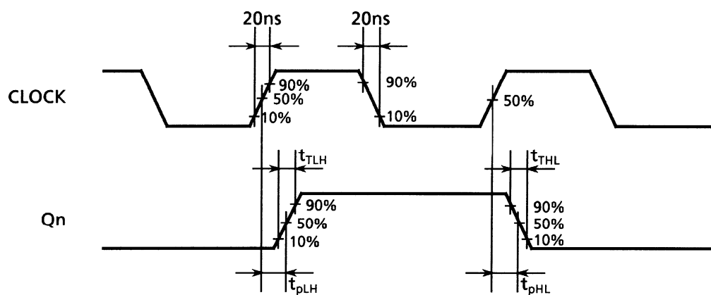
波形 1
