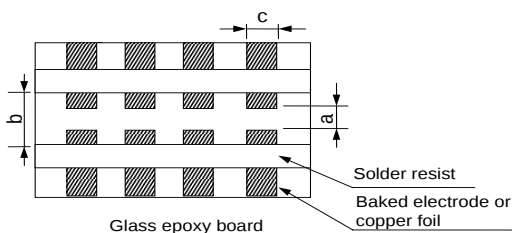
Fig.3 (in:mm)
