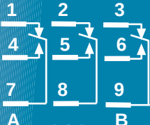
3PDT
