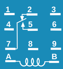
SPDT
