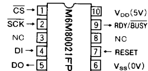
Outline 10P2N-A
