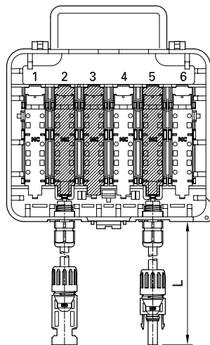
PV-JB/S2-2/N2,5SXL/... PV-JB/S2-2/N4SXL/...
