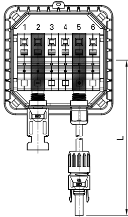
PV-JB/2-1/N...
