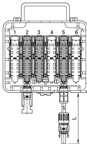
PV-JB/S2-1/N2,5SXL/... PV-JB/S2-1/N4SXL/...
