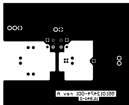
Figure 44. Bottom Layer
