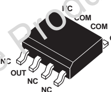
SO-8 ACS102-5T1
