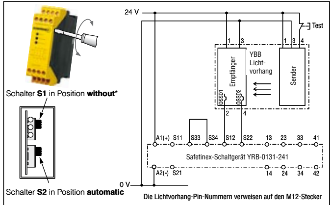
FIG. 41: AUTOMATISCHER START
