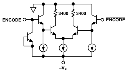
AD9027 Encode Input
