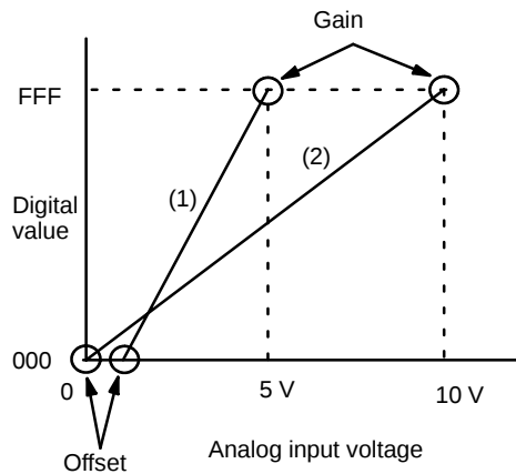
Voltage Inputs
