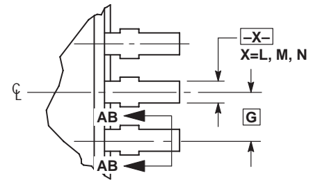
VIEW Y
