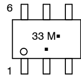
SOT-363 CASE 419B-02
