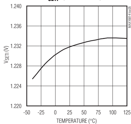
VSETI vs. TEMPERATURE
