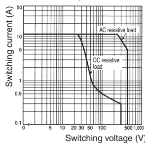
G2RL-1A, G2RL-1
