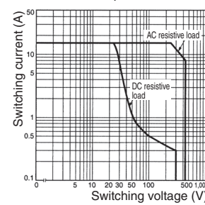
G2RL-1A-E, G2RL-1-E
